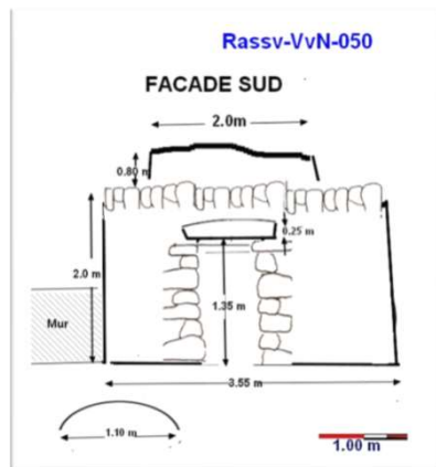
CABANE N°50 PARCELLE 593 QUARTIER PALLAIS/FONT DE L'AUBE Linteau monolithique en plein cintre en pierre de taille.
